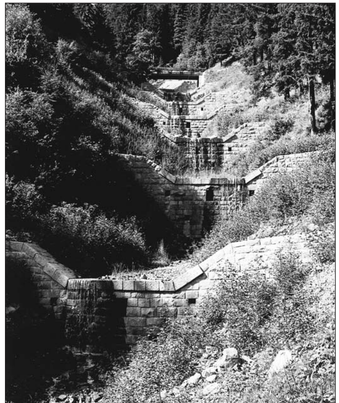
Vier Jahre später: Der Vergeinbach ist verbaut, die Uferböschungen sind wieder bewachsen. Der Wildbach hat viel von der bedrohlichen Gefährlichkeit verloren.
